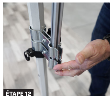
ÉTAPE 12 Insérer les mâts dans les connecteurs en les maintenant alignés.
