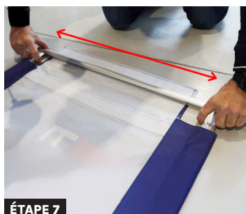
ÉTAPE 7 Ajuster l'espace entre les barres pour bien tendre la bâche.
